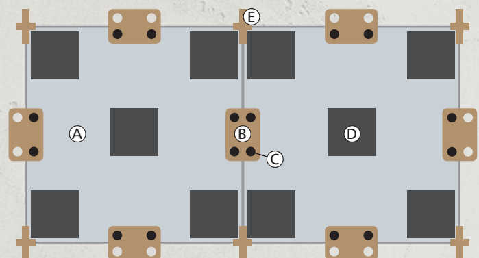
Ansicht Unterseite | bottom side view
